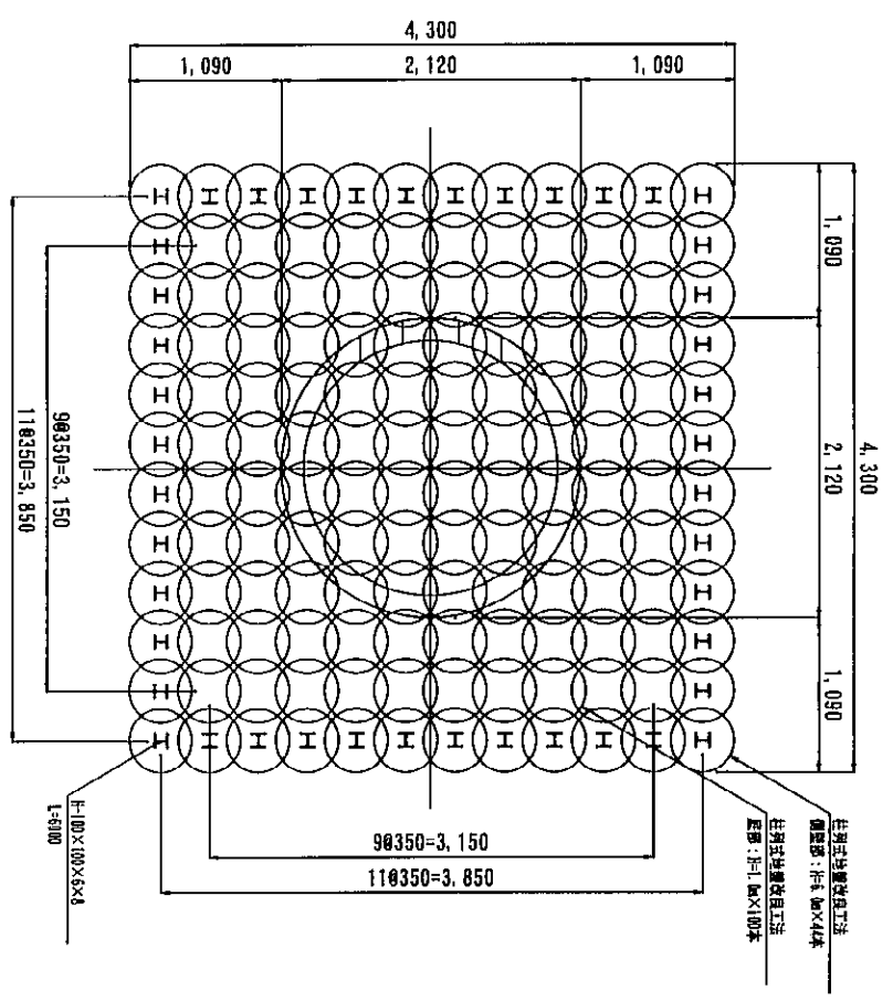
下部平面図 S=1/30
